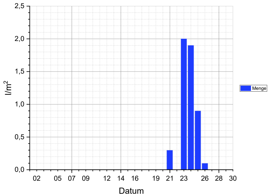
Tagesniederschlag April 2025
