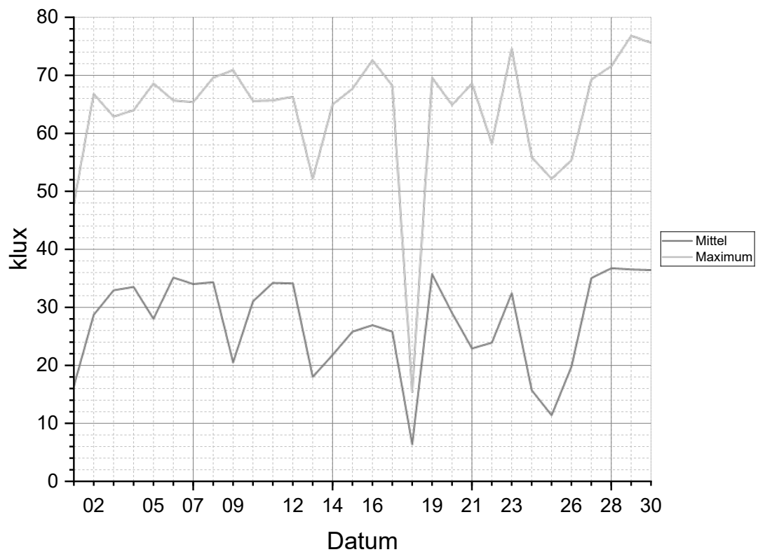
Tageshelligkeit April 2025
