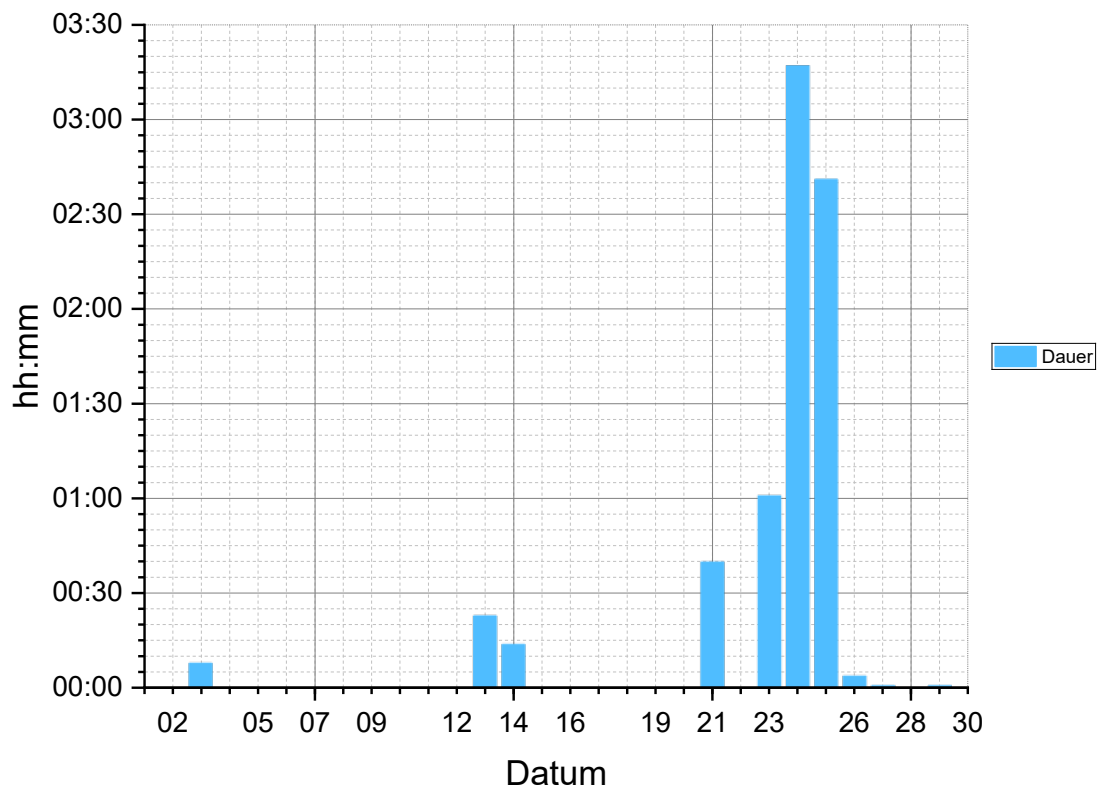
Tagesniederschlag April 2025
