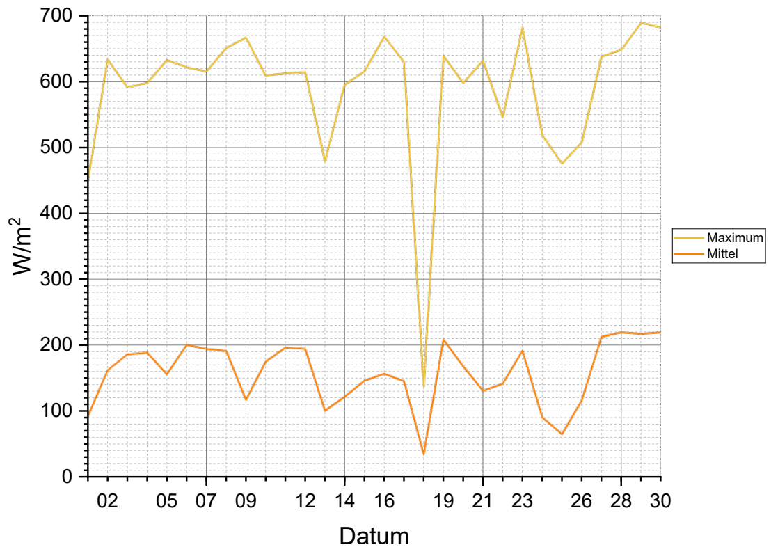
Tagesglobalstrahlung April 2025
