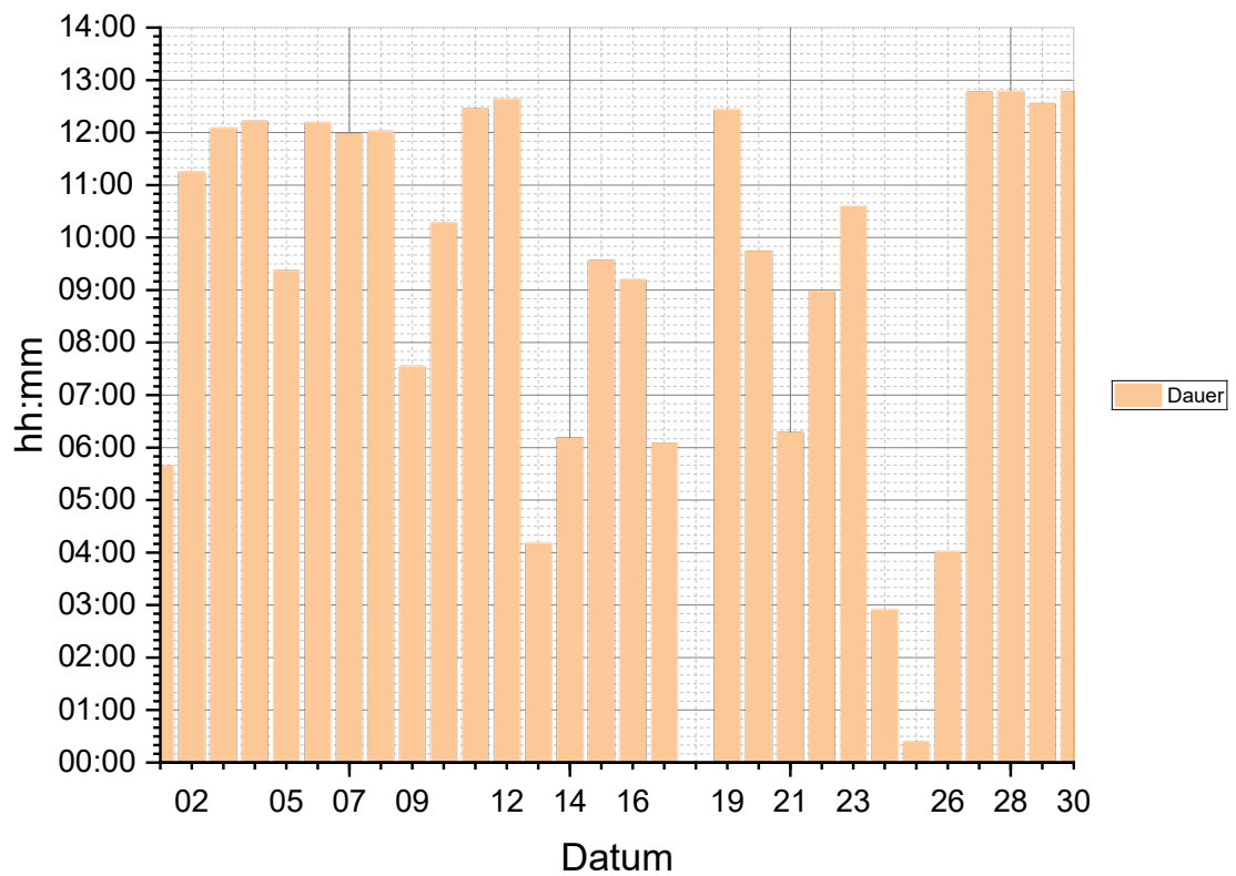
Tagessonnenschein April 2025
