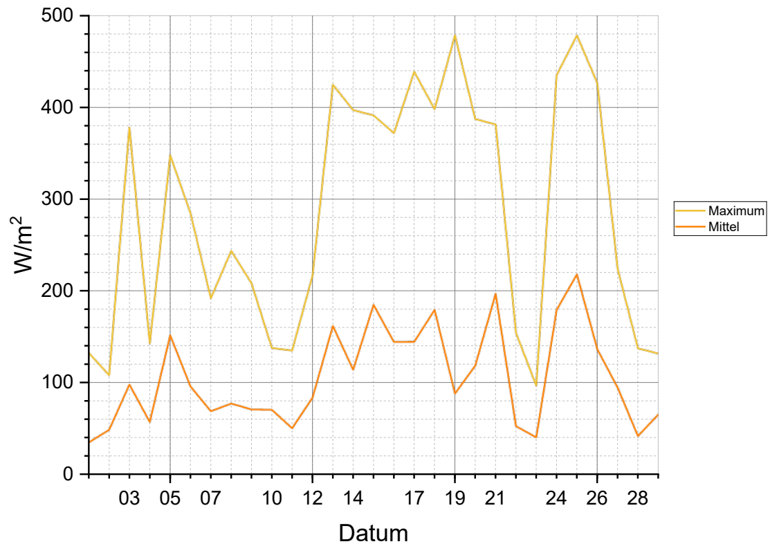
Tagesglobalstrahlung Februar 2024
