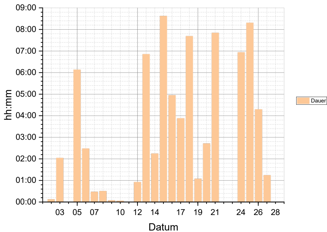
Tagessonnenschein Februar 2024
