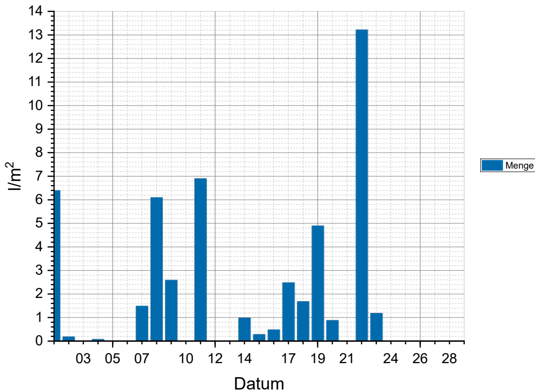
Tagesniederschlag Februar 2024
