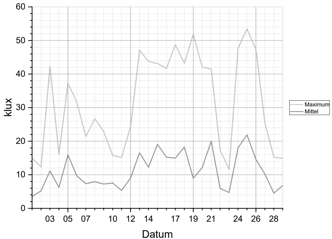
Tageshelligkeit Februar 2024
