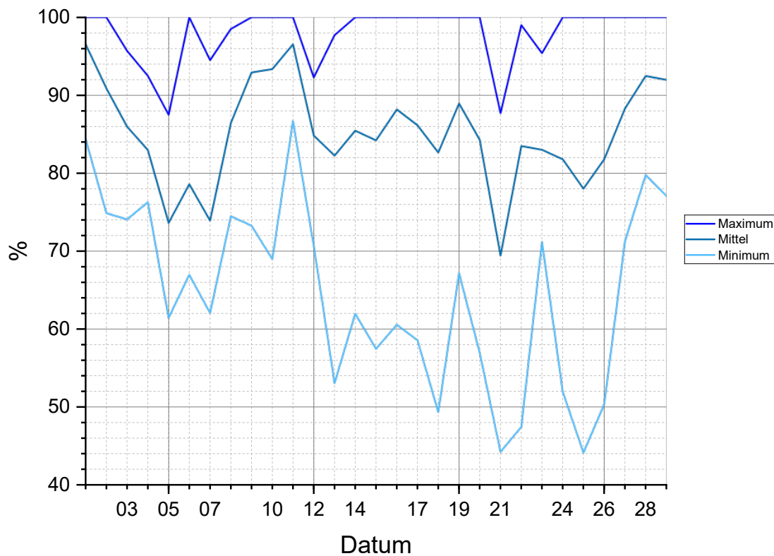
Tagesluftfeuchtigkeit Februar 2024
