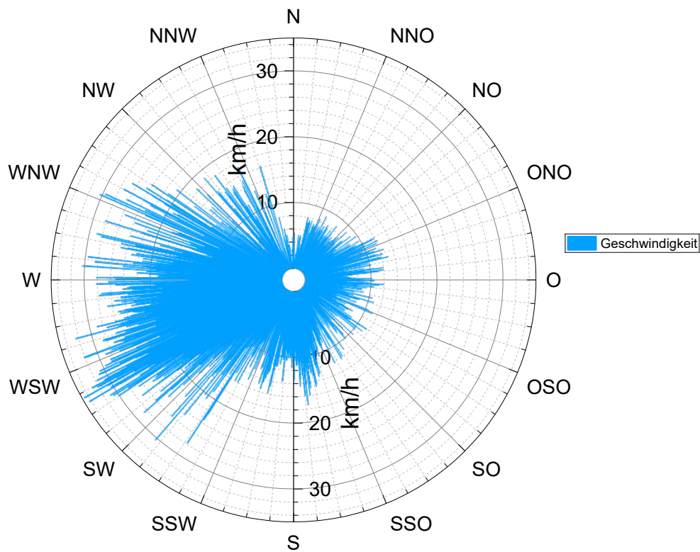
Wind-Maximum Februar 2024
