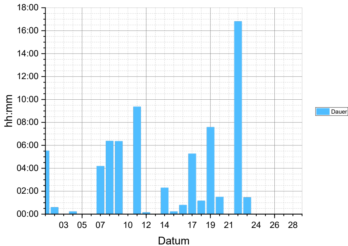
Tagesniederschlag Februar 2024
