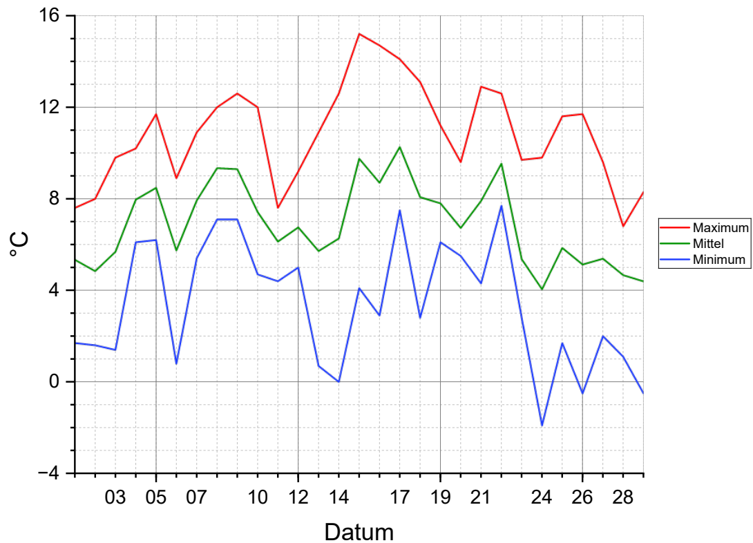
Tageslufttemperatur Februar 2024
