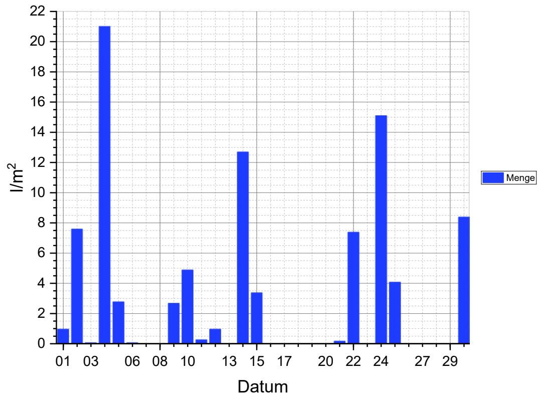
Tagesniederschlag September 2025
