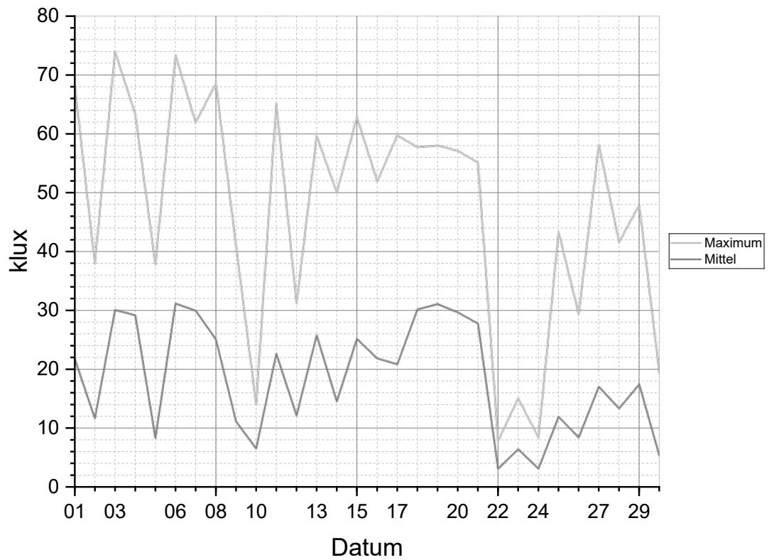
Tageshelligkeit September 2025
