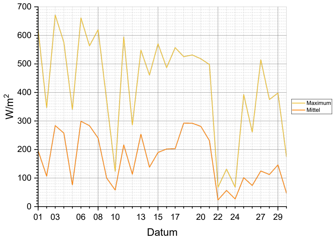
Tagesglobalstrahlung September 2025
