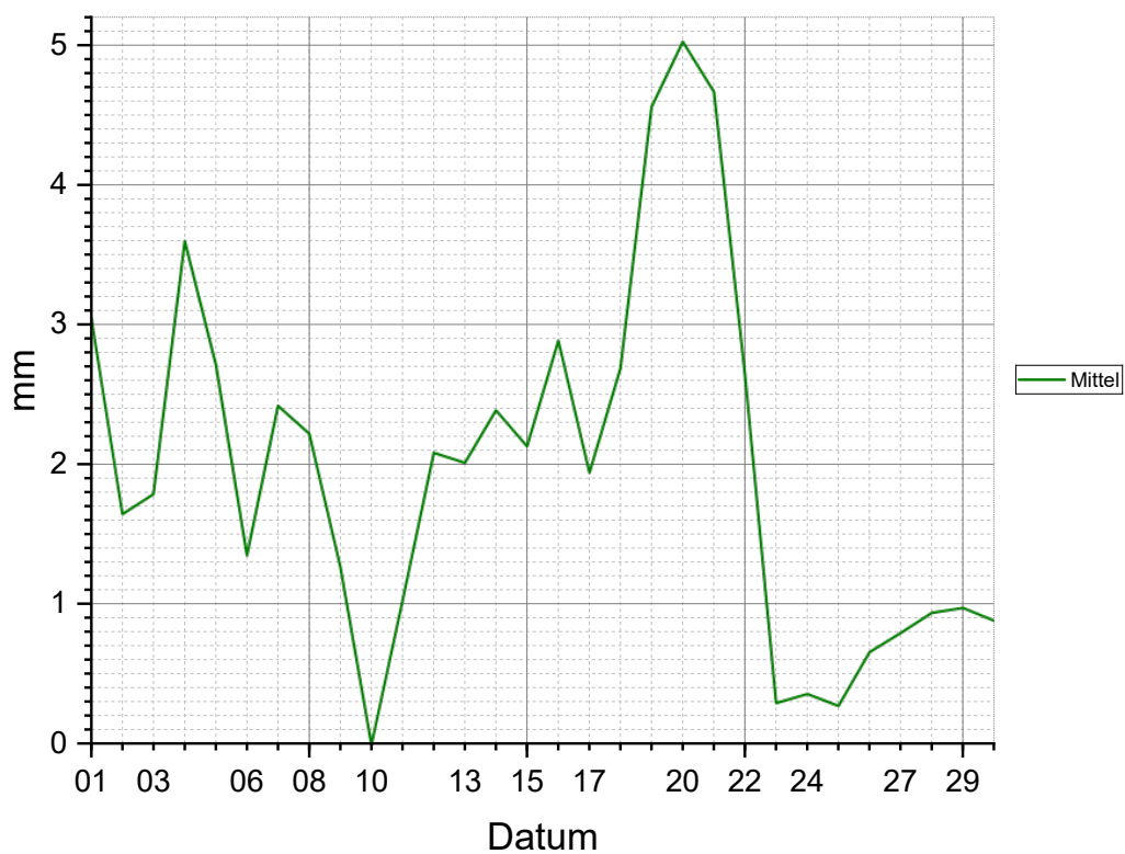
Tagesverdunstung September 2025
