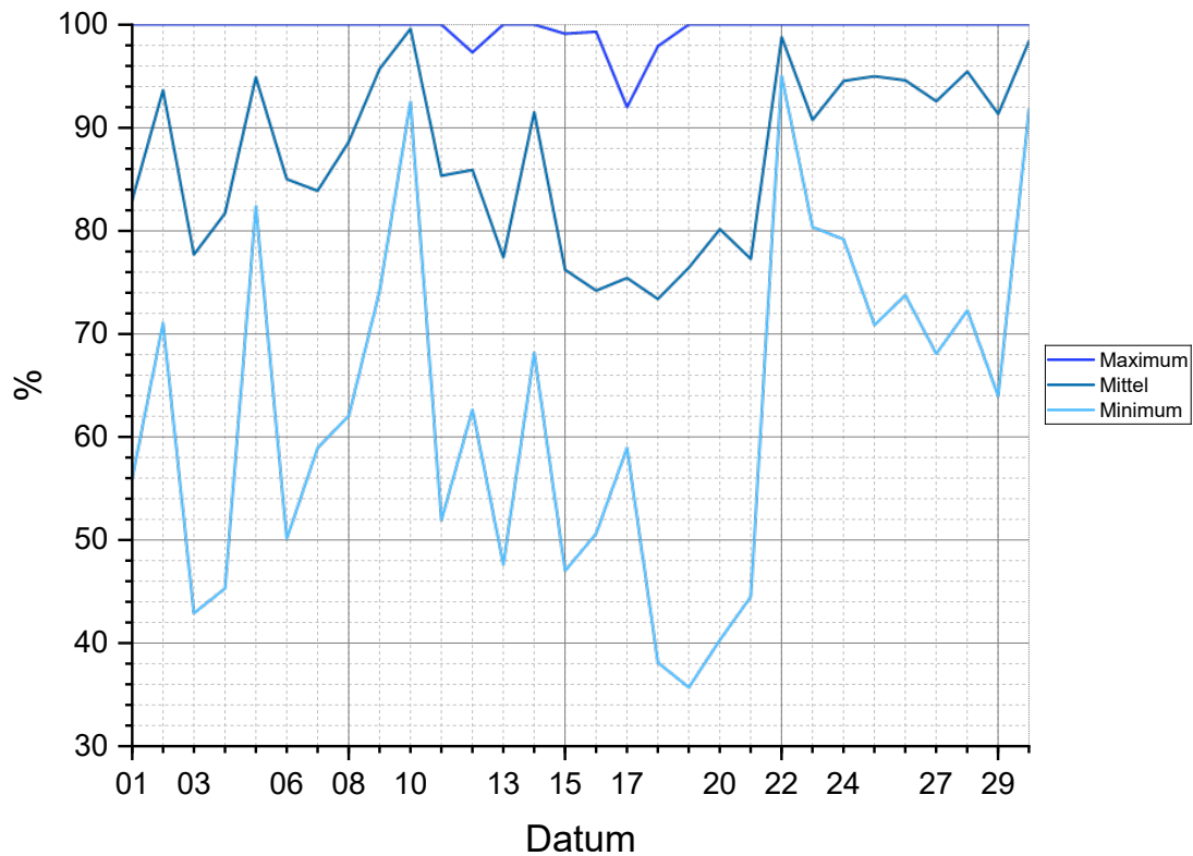
Tagesluftfeuchtigkeit September 2025
