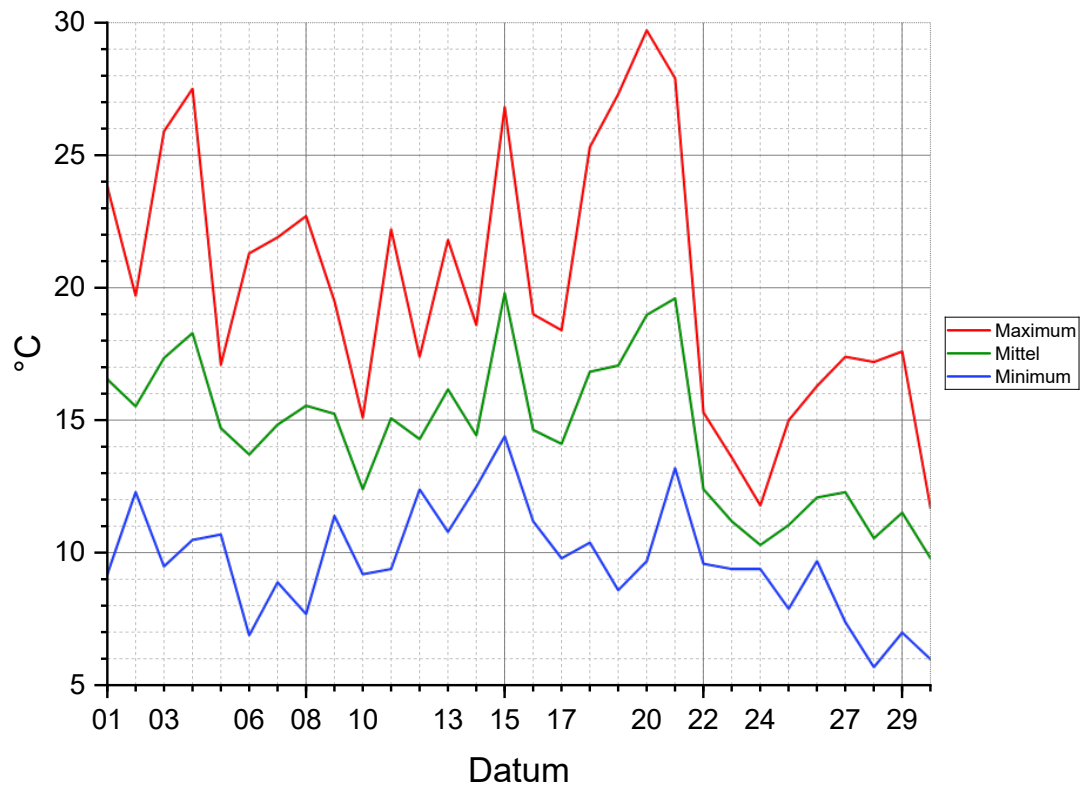
Tageslufttemperatur September 2025
