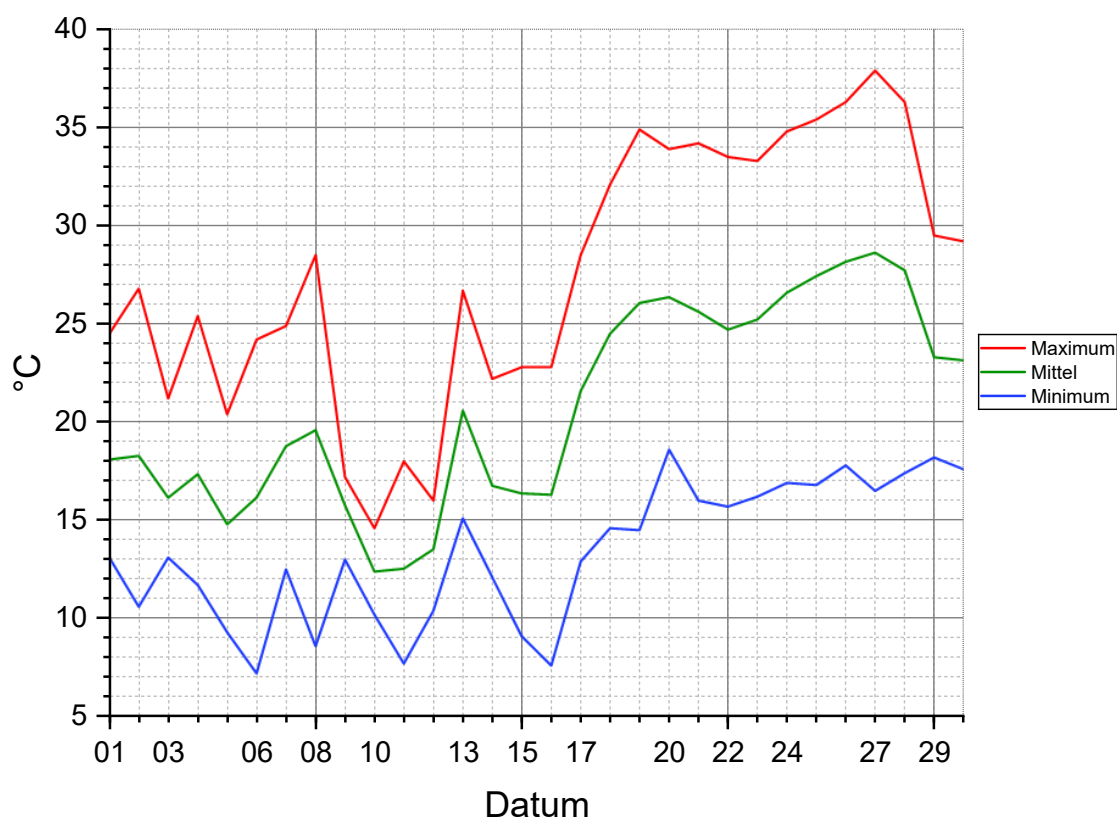
Tageslufttemperatur Juni 2026
