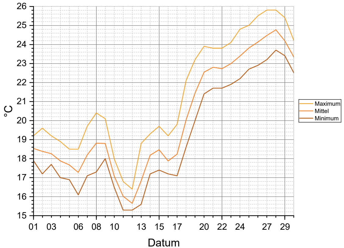
Tagesbodentemperatur Juni 2026
