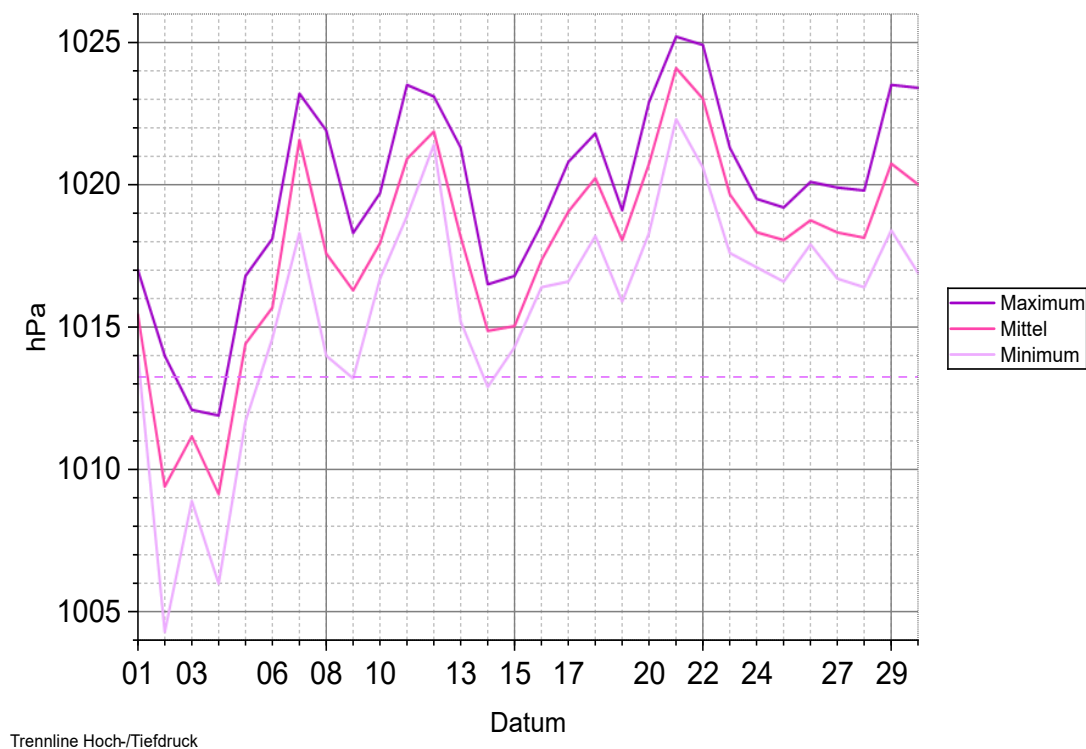
Tagesluftdruck Juni 2026
