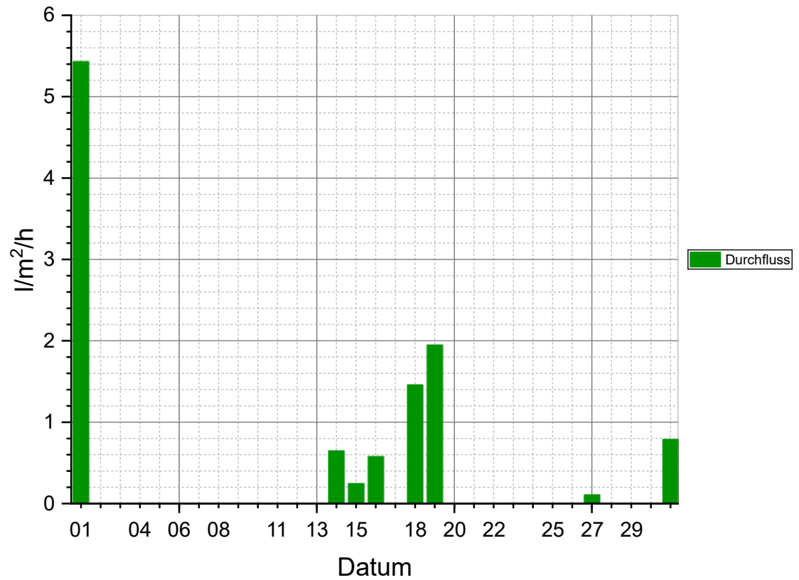
Tagesniederschlag Juli 2026
