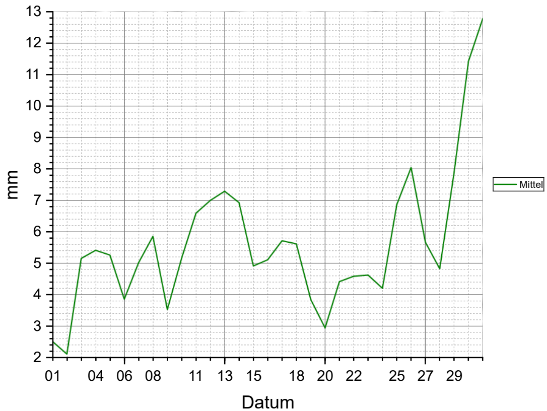
Tagesverdunstung Juli 2026
