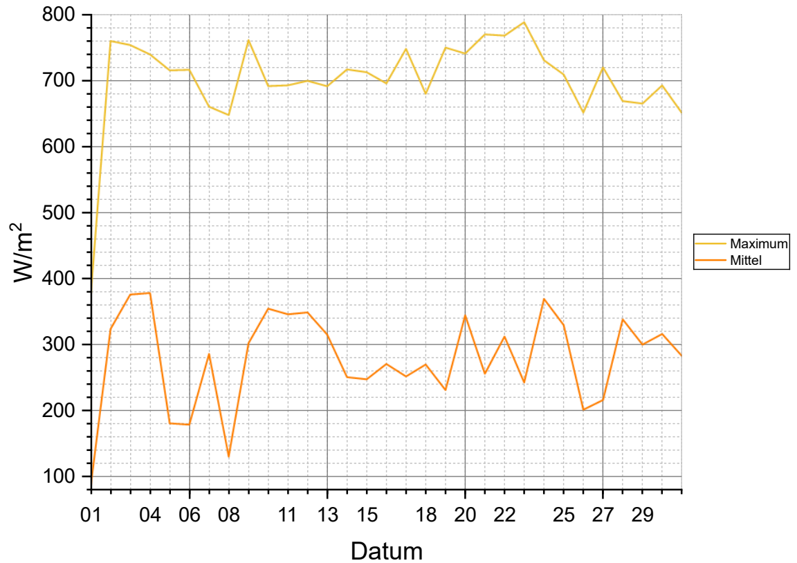
Tagesglobalstrahlung Juli 2026
