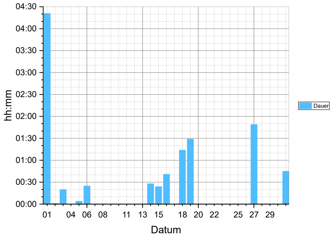
Tagesniederschlag Juli 2026
