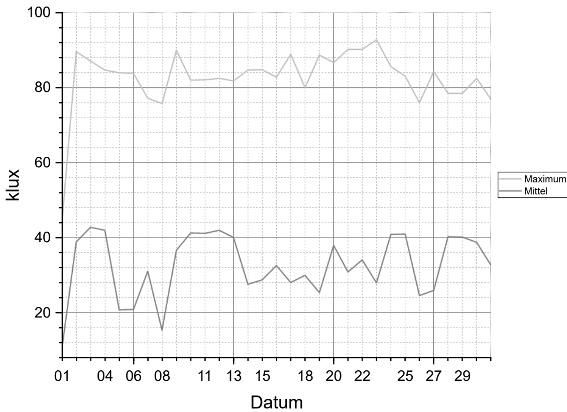
Tageshelligkeit Juli 2026
