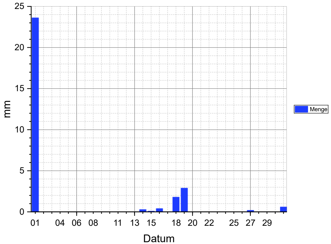
Tagesniederschlag Juli 2026
