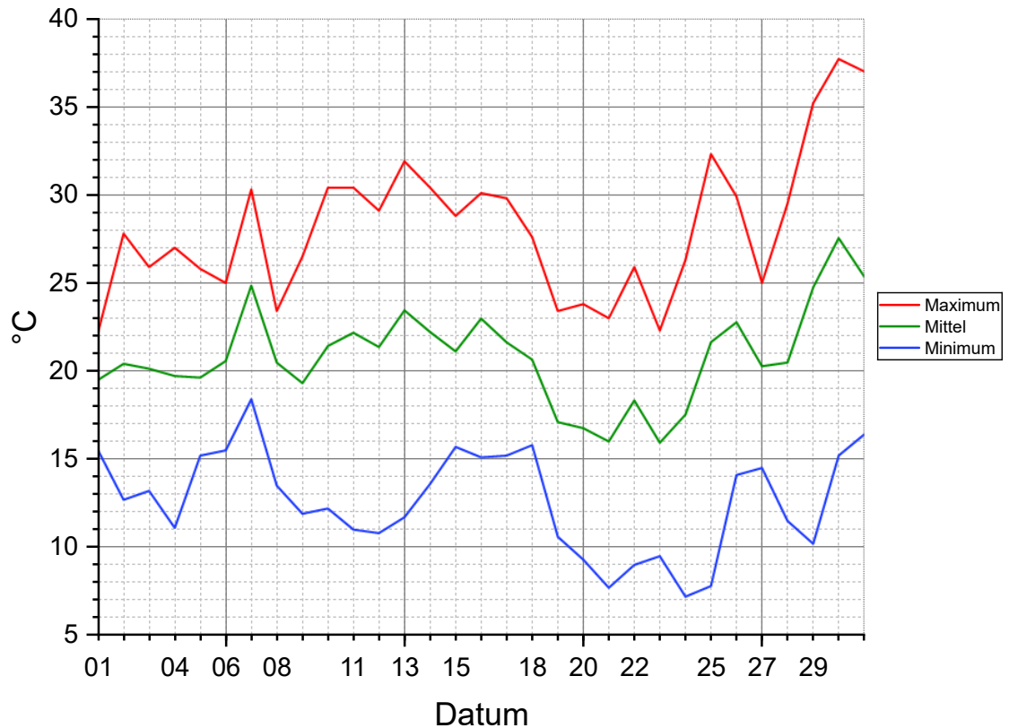
Tageslufttemperatur Juli 2026
