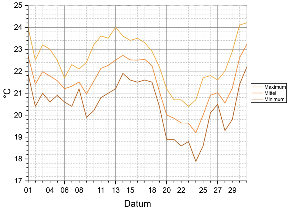
Tagesbodentemperatur Juli 2026
