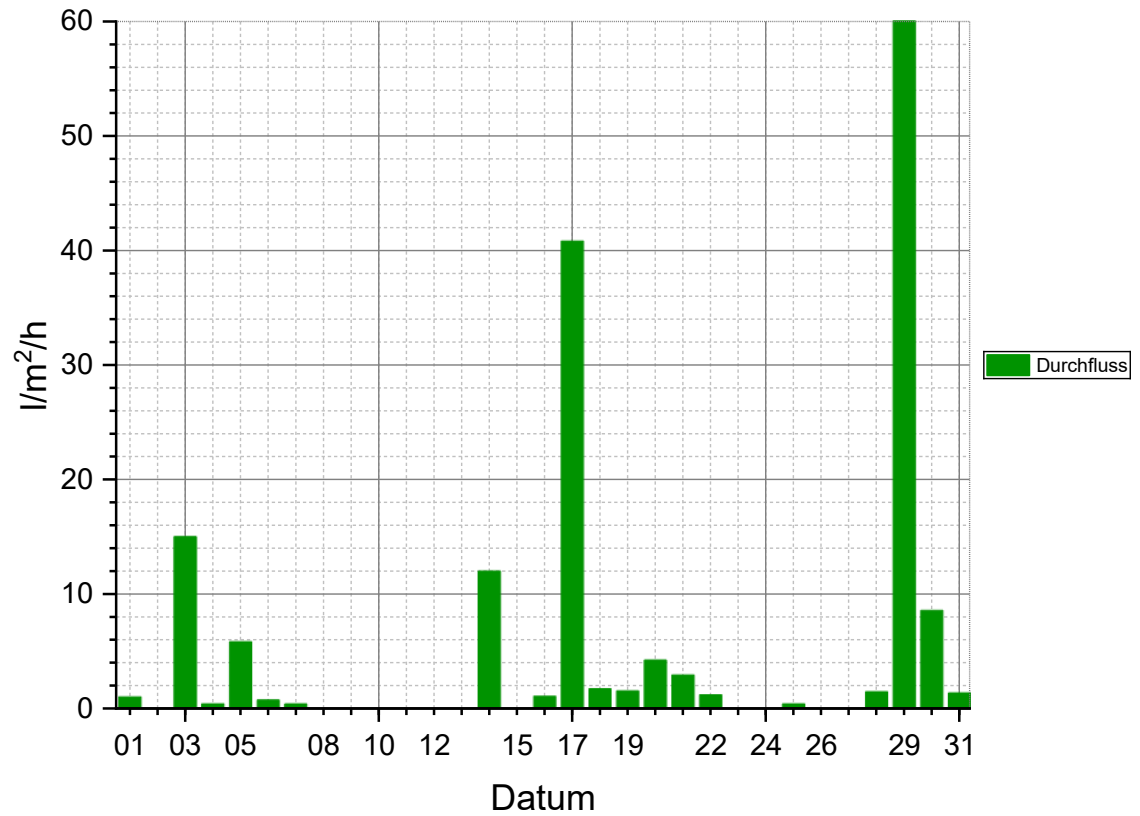
Tagesniederschlag August 2026
