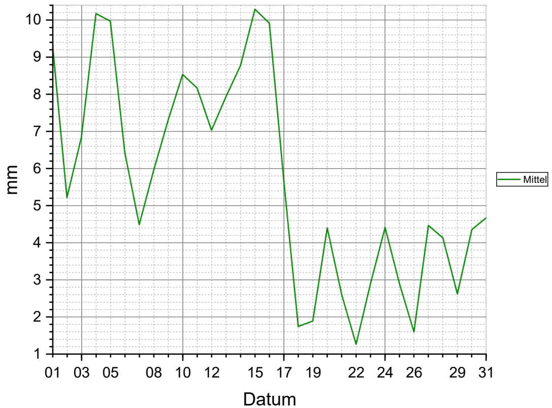
Tagesverdunstung August 2026
