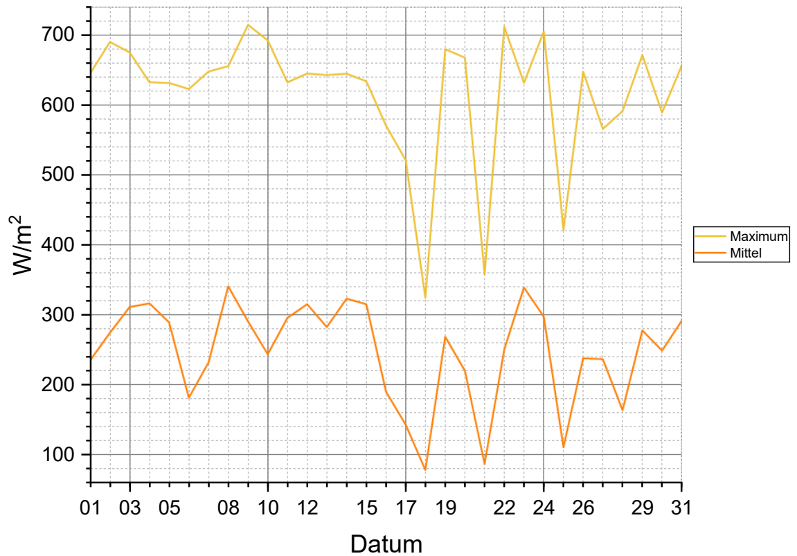
Tagesglobalstrahlung August 2026
