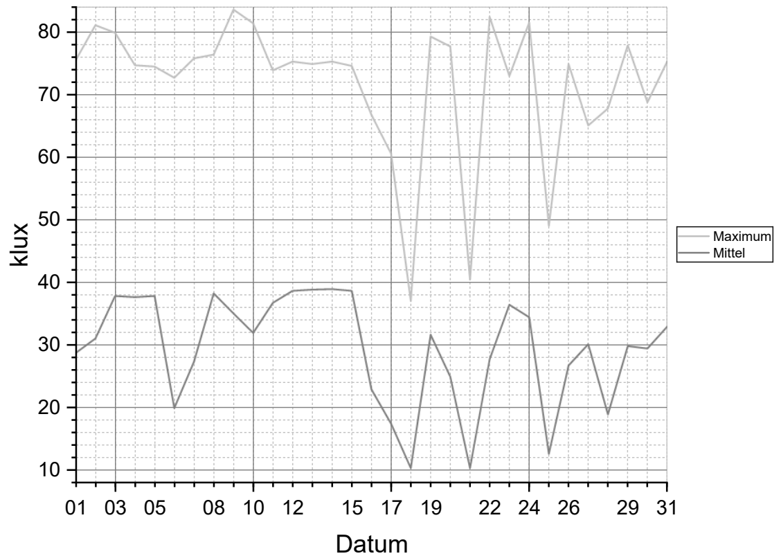
Tageshelligkeit August 2026
