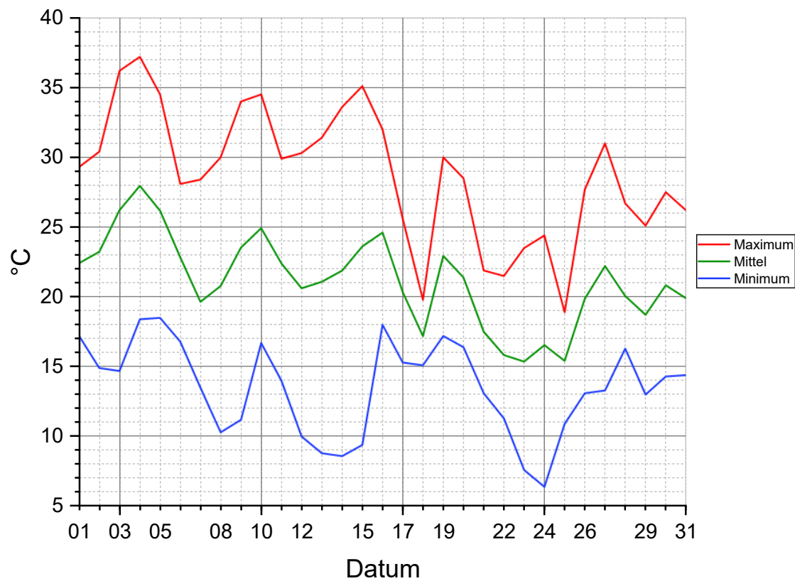
Tageslufttemperatur August 2026
