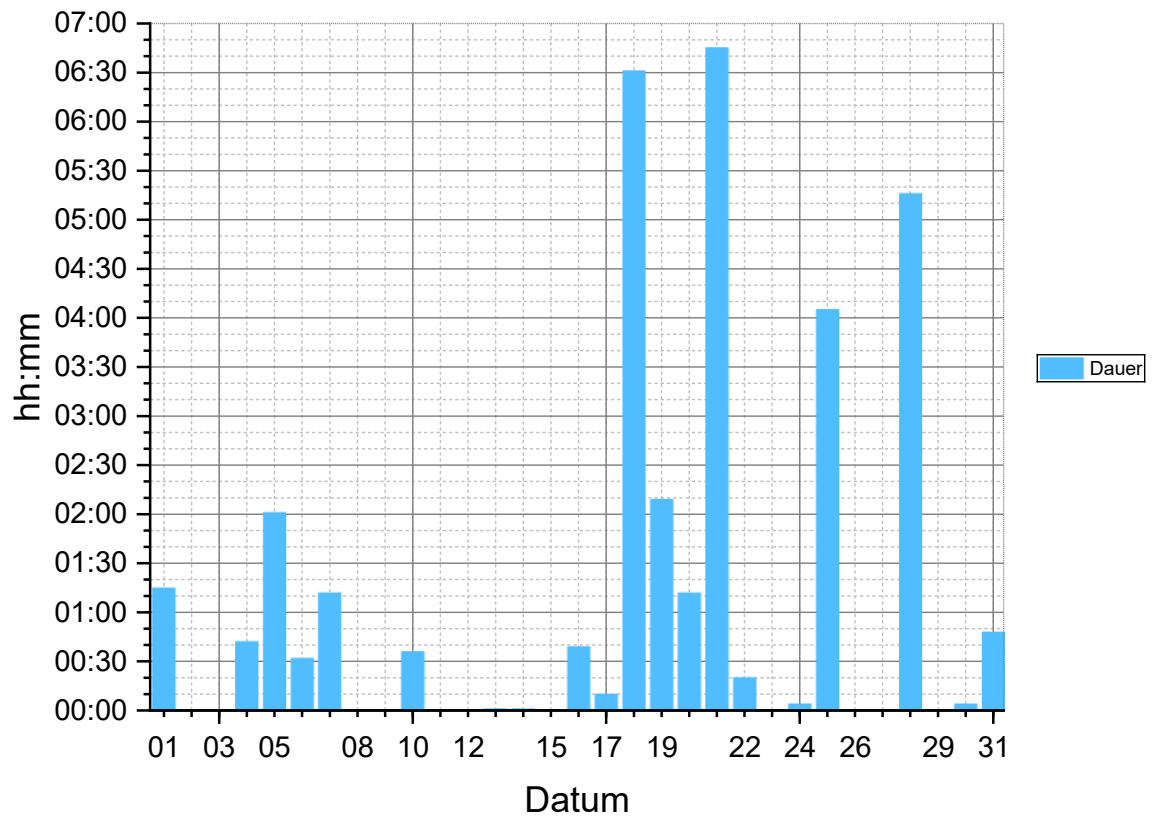
Tagesniederschlag August 2026
