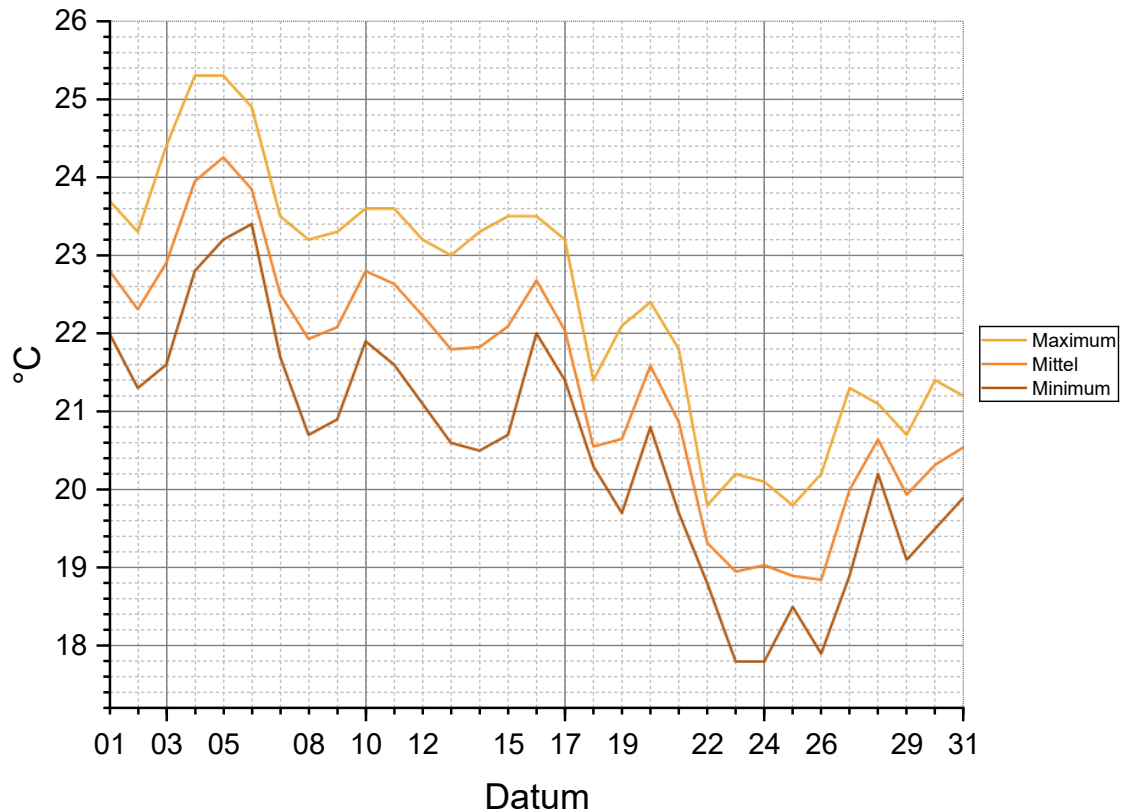
Tagesbodentemperatur August 2026
